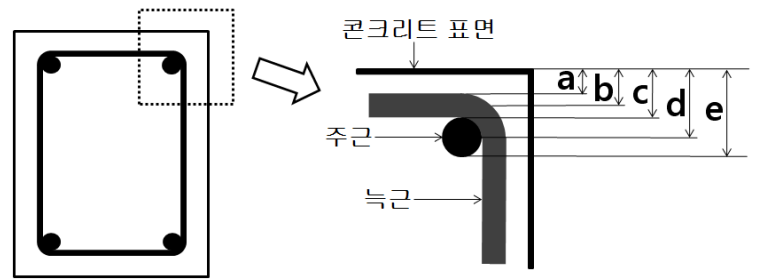
<철근콘크리트보 단면 및 상세>
